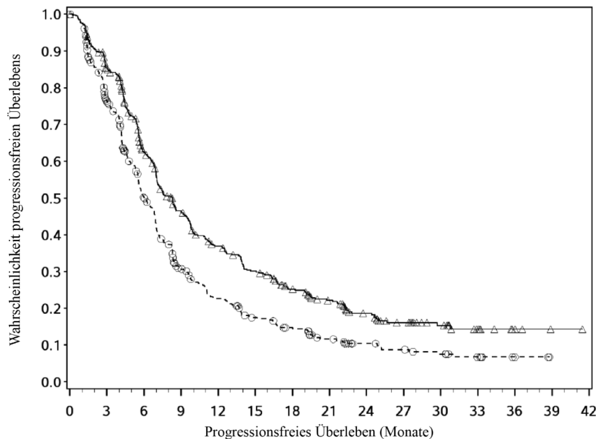
Abbildung 31: Kaplan-Meier-Kurven des progressionsfreien Überlebens bei Patienten mit PD-L1 CPS \geq 5 (CA209649)
