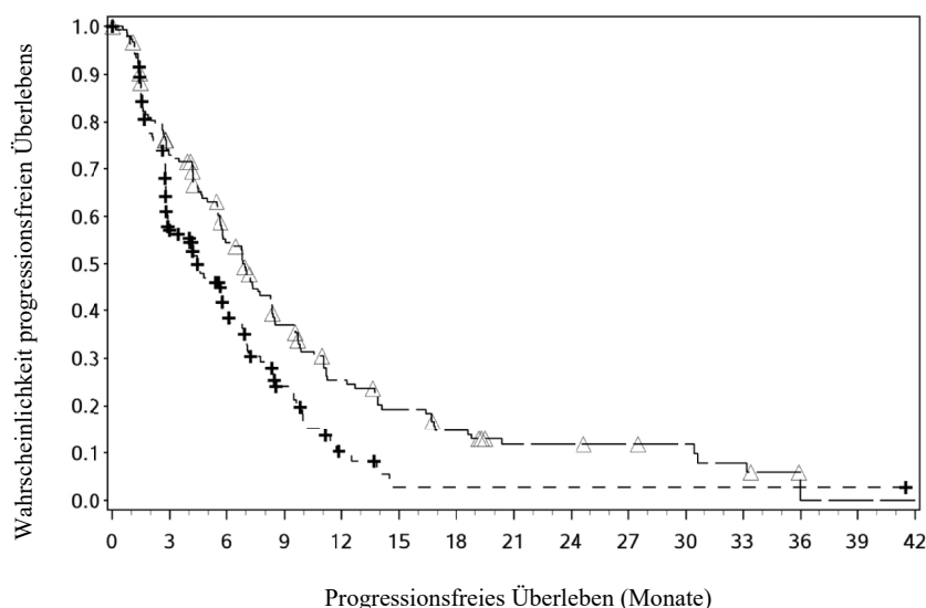
Abbildung 28: Kaplan-Meier-Kurven des PFS bei Patienten mit Tumorzell-PD-L1 \geq 1\% (CA209648)
