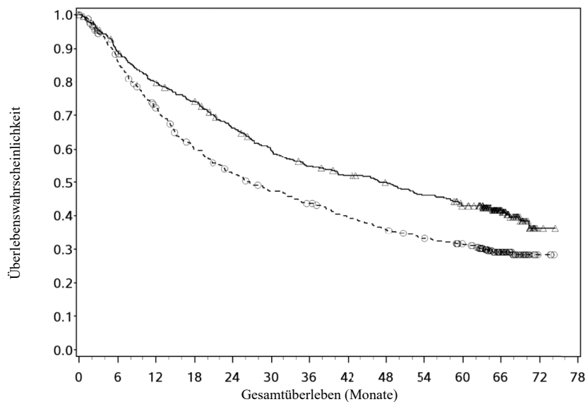
Abbildung 18: Kaplan-Meier-Kurven des Gesamtüberlebens bei Patienten mit intermediärem/ungünstigem Risikoprofil (CA209214) – Minimale Nachbeobachtungszeit 60 Monate
