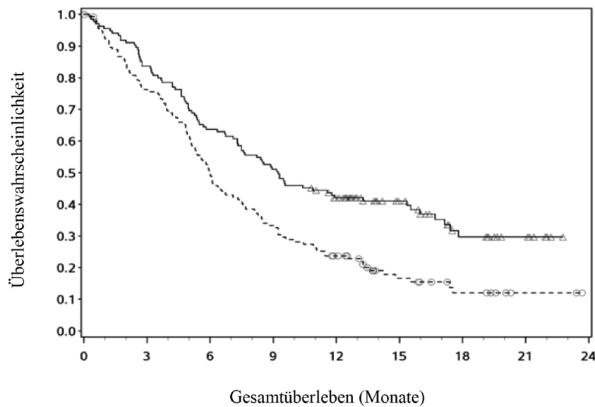
Abbildung 14: Kaplan-Meier-Kurven des Gesamtüberlebens (CA209017)
