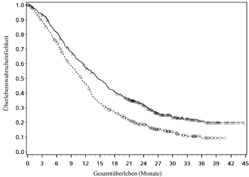
Abbildung 30: Kaplan-Meier-Kurven des Gesamtüberlebens bei Patienten mit PD-L1 CPS \geq 5 (CA209649)
