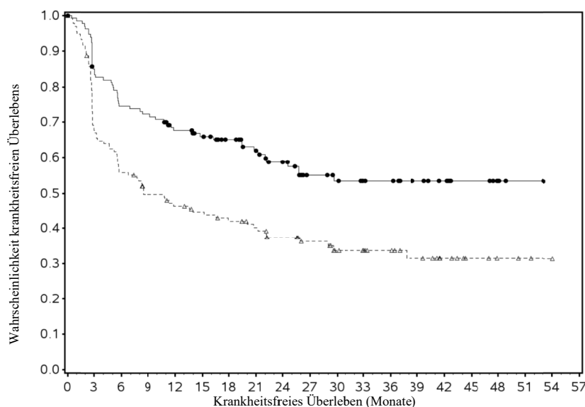
Abbildung 24: Kaplan-Meier-Kurven des DFS bei Patienten mit Tumor-PD-L1-Expression \geq 1\% (CA209274)
